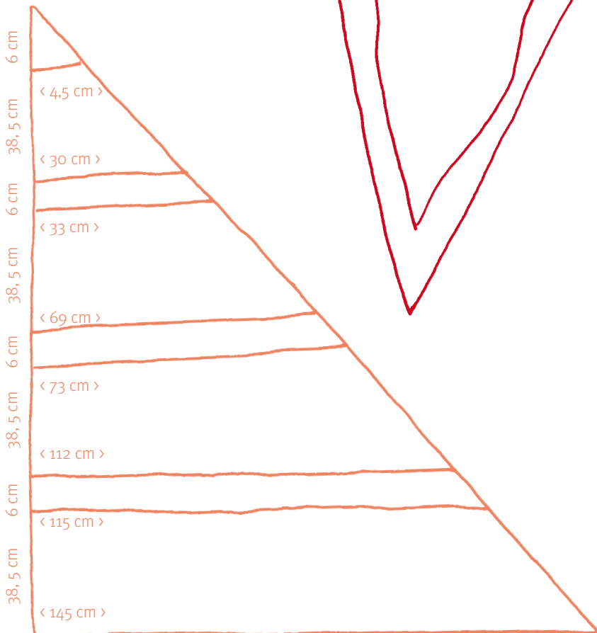
Maße für den Baldachin (inkl. Nahtzugabe)
